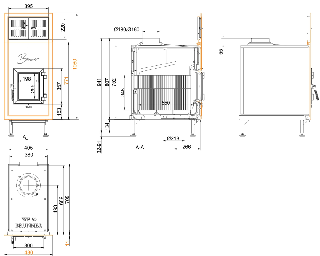
... Gussfrontplatte 1060 x 480
