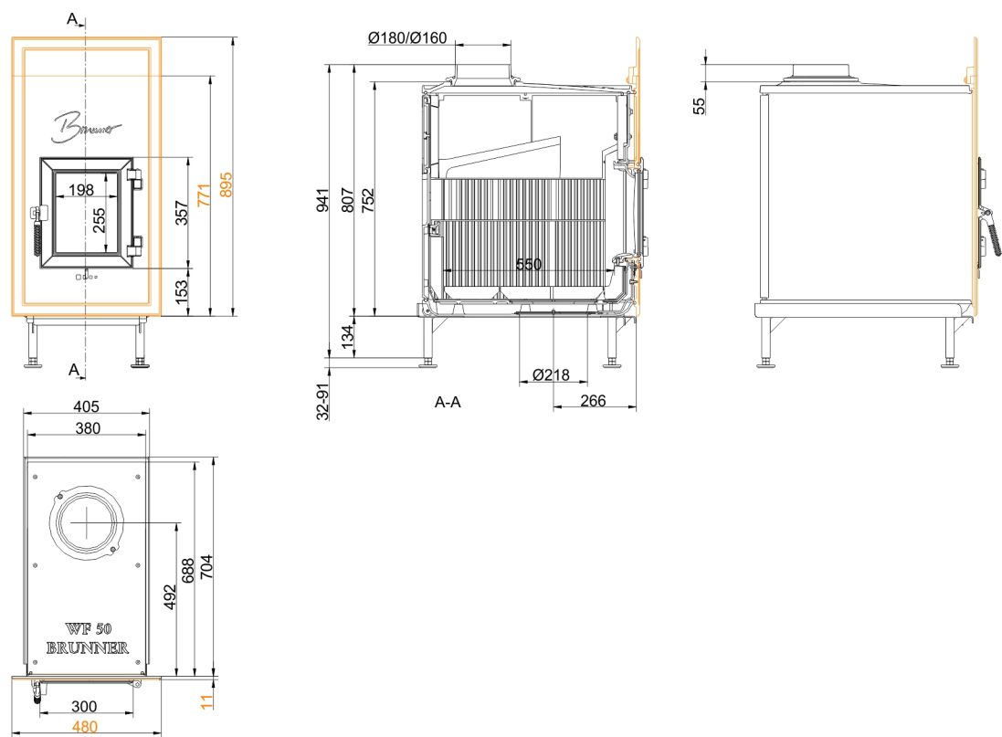
... Gussfrontplatte 895 x 480
